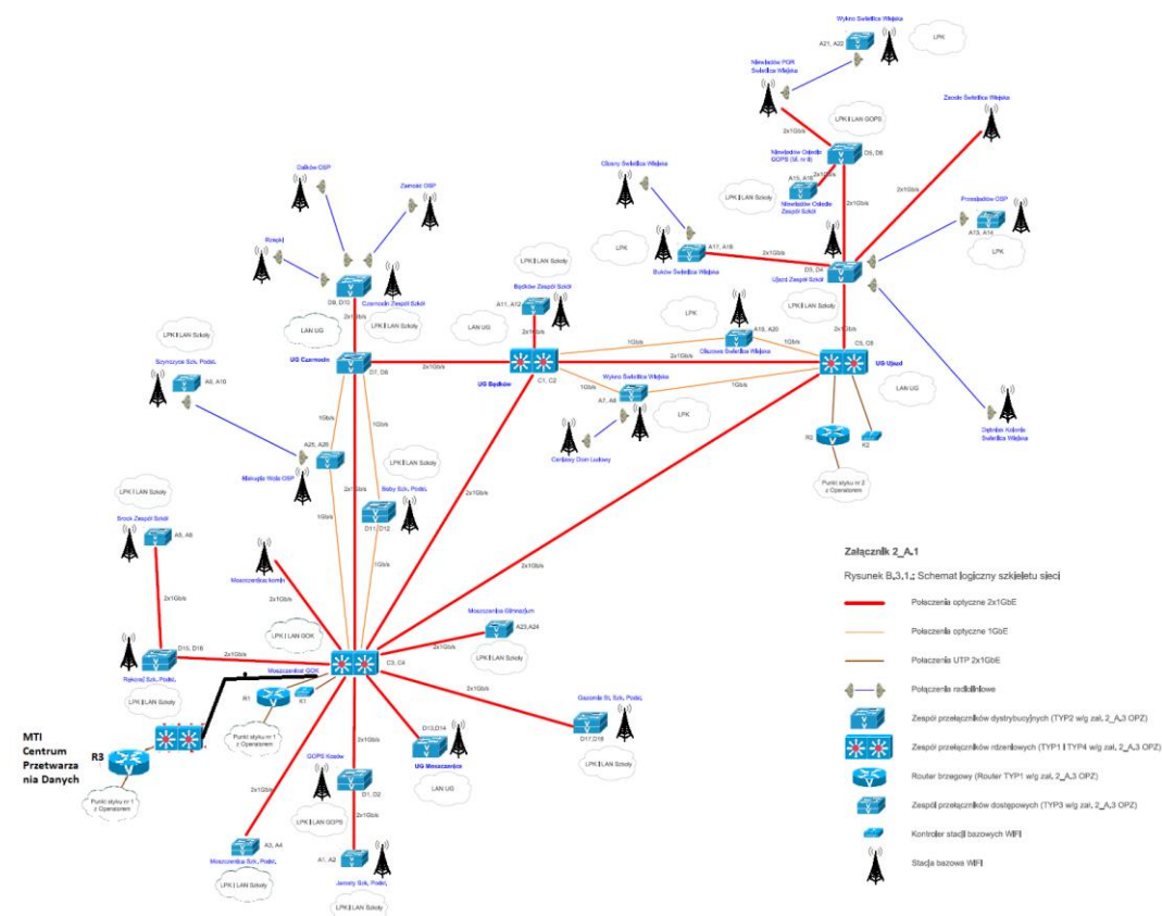
Rysunek 2. Schemat infrastruktury konsorcjum gmin E-leader.
